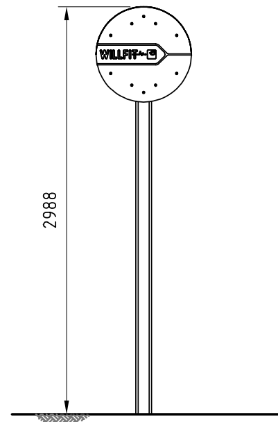
Elevation
