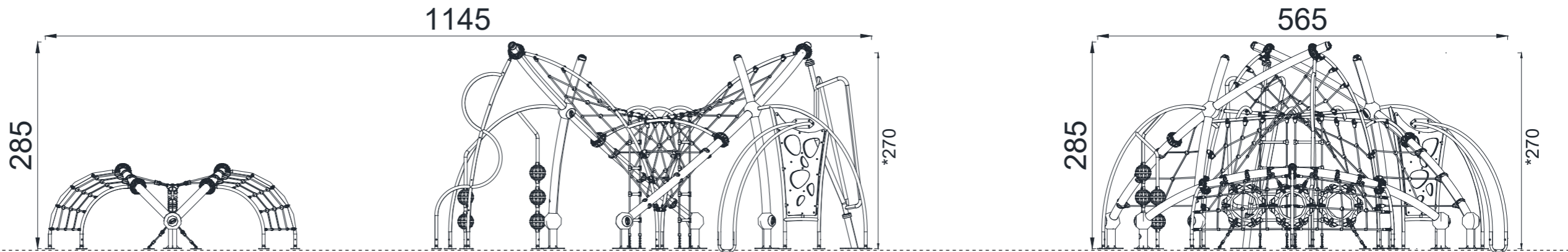
ÖN GÖRÜNÜŞ / FRONT VIEW
